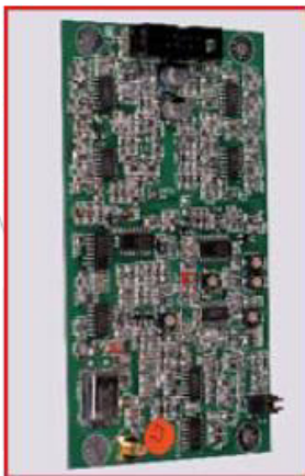
Stereo Encoder
